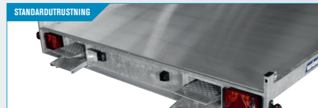
Alufflakbotten i kraftig konstruktion. Halsksäker och stark. Uppköringsramper förvaras i rampfack under flaket. 2,5 m - 4.000 kg
