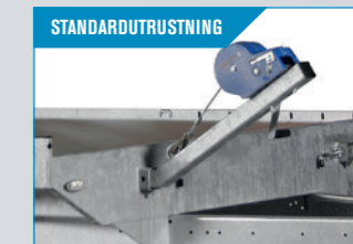
Vajervinsch. När bilar och maskiner skal vinschas upp på flaket. El-vinsch kan köpas.
