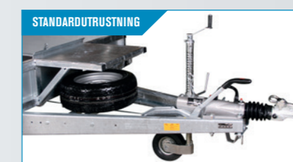
Skopstöd, reservhjul och stödhjul är standard.
