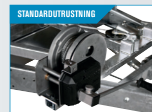
STANDARDUTRUSTNING Vajerwinsch. När fordon ska vinschas upp på flaket.
